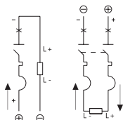
Рис. 1 e.mcb.stand.60.DC.1-63
