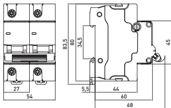
Рис. 4 e.mcb.stand.60.DC.125
