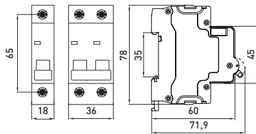
Рис. 3 e.mcb.stand.60.DC.1-63
