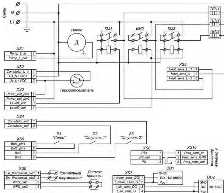
Схема электрическая принципиальная котла Tenko «Standart Digital+». Напряжение питания котла- 380В, Напряжение питания ТЭН -380В.
