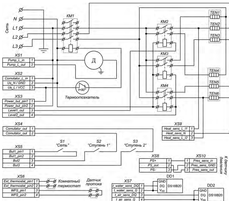
Схема электрическая принципиальная котла Tenko «Standart Digital+». Напряжение питания котла- 380В, Напряжение питания ТЭН -380В, 2 блока Скачано с сайта интернет магазина https://axiomplus.com.ua/
