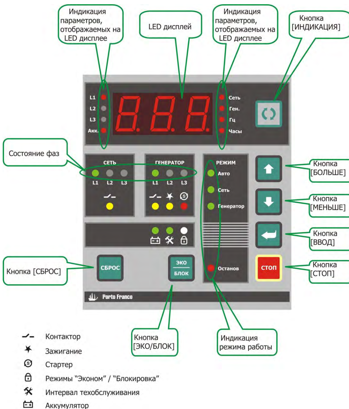
Рис. 5.2. Панель индикации и управления
