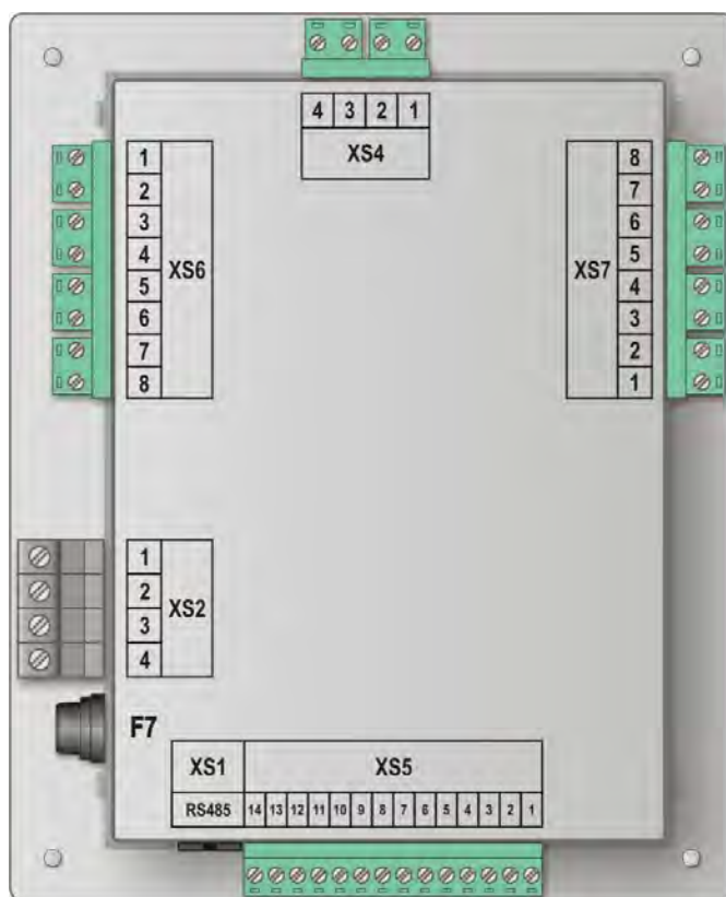
Рис 6.1. Клеммы и разъёмы подключения контроллера (вид сзади).
