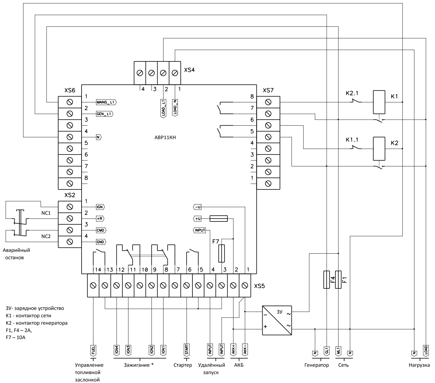
Рис 6.2. Пример схемы подключения контроллера АВР11КН.
