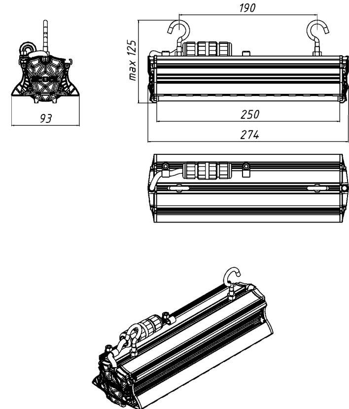
Рисунок 1 Светильник «L-industry 30 Turbine» с подвесным креплением.
