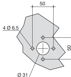
Монтажное отверстие
