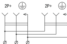
Рисунок 3 – Электрическая схема соединений РБ32-1-0м
