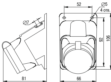
Рисунок 13 – Розетка с защитной крышкой угловая настенная РБУ13-1-0м
