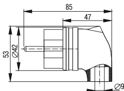
Рисунок 7 – Вилка с боковым вводом ВБу3-1-0м
