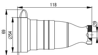
Рисунок 6 – Вилка прямая ВБп3-1-0м
