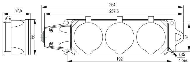
Рисунок 11 – Розетка (колодка) трёхместная с защитными крышками РБ33-1-0м
