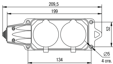
Рисунок 10 – Розетка (колодка) двухместная с защитными крышками РБ32-1-0м
