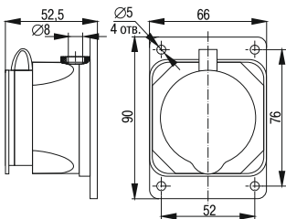
Рисунок 9 – Розетка с защитной крышкой настенная РБ13-1-0м
