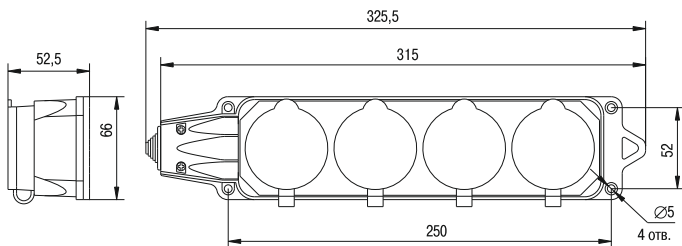
Рисунок 12 – Розетка (колодка) четырехместная с защитными крышками РБ34-1-0м
