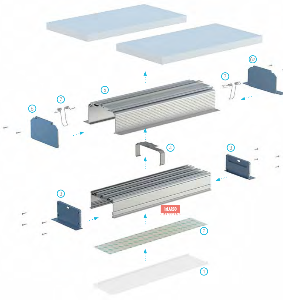
Explosionszeichnung zum Beleuchtungssystem bestehend aus folgenden Elementen: Profil inLARGO, (1) Abdeckung SUPER WIDE, (2) LED-Streifen, (3) Endkappen inLARGO mit Öffnung, (4) Zwischenprofil-Verbinder LARGO, (5) Montageprofil LARGO M3, (6) Endkappe LARGO M3 mit einfachem Finish, (6a) Endkappe LARGO M3 mit vollem Finish, (7) Montagefedern
