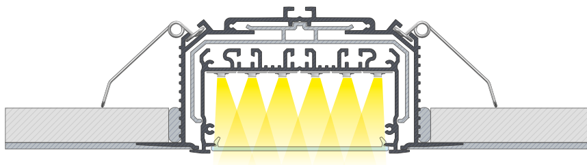
Fertiges Resultat nach der Montage des Profilsystems inLARGO mit Abdeckung SUPER WIDE, Zwischenprofil-Verbinder LARGO, Montageprofil LARGO M3 und Montagefedern mit verputztem Teil des Profils
