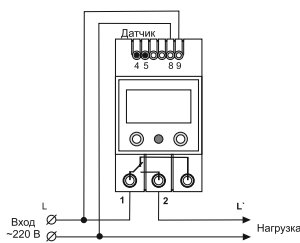
Схема подключения
