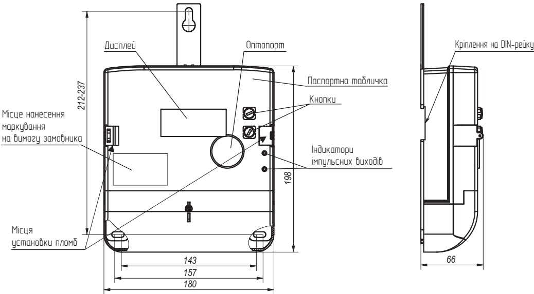
Малюнок А.1 - Загальний вигляд, габаритні і установчі розміри, місця установки пломб на корпусі трифазного лічильника прямого включення типу MTX 3...0.D...4...3-...4
