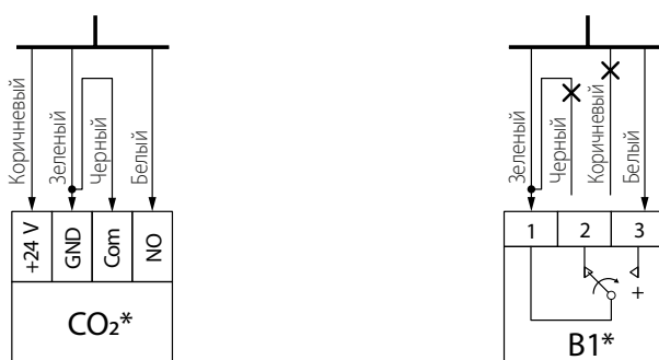
Схема подключения датчика влажности или CO 2 внутри установки
