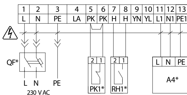
Схема подключения датчика влажности или CO 2 внутри установки
