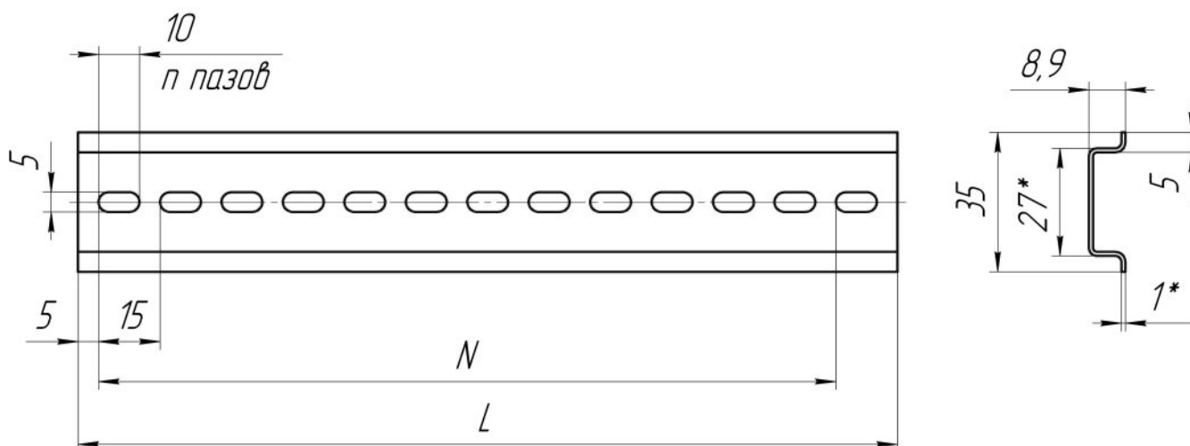
Габаритные размеры DIN-рейки
