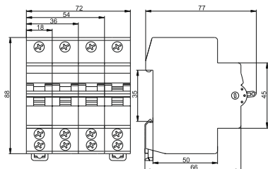
Размеры для исполнений I_e = 50; 63 \text{ A}
