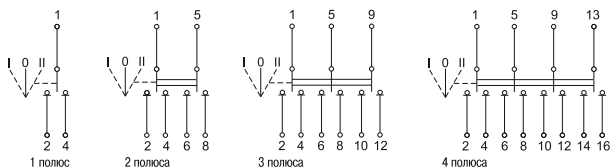
Рисунок 2 – Схемы электрические выключателя
