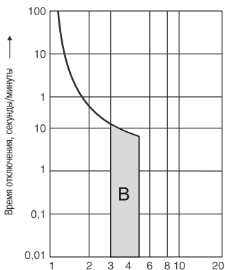
Рисунок 1. Времятоковые характеристики срабатывания ВА47-60 от сверхтока. Тип B
