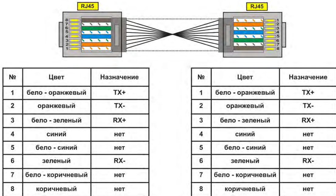
Рисунок 5.3 – Нумерация выводов кабеля соединения с сетью Ethernet
