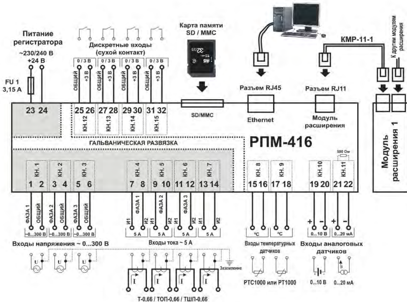
FU1 – Предохранитель (автоматический выключатель) на ток 3,15 А
