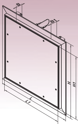
Ревизионные дверцы для монтажа в конструкции из гипсокартона
