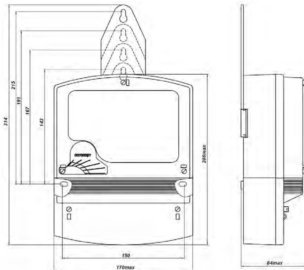
Рисунок 2 - Габаритні і присьднувальні розміри лічильника
