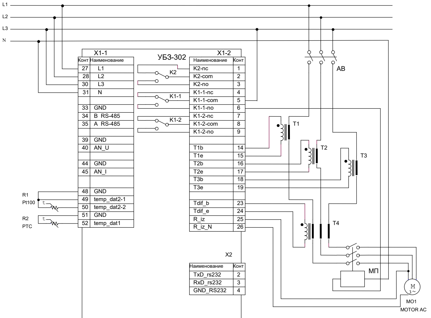
Рисунок 2.1 - Схема подключения УБЗ
