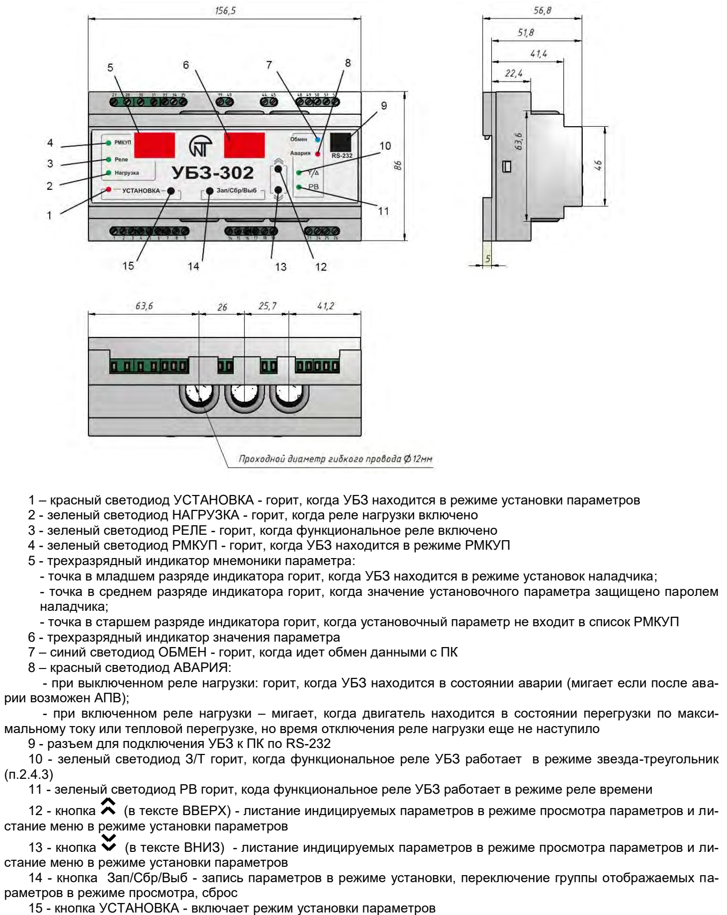
Рисунок 1.1 - Органы управления и габаритные размеры УБЗ
