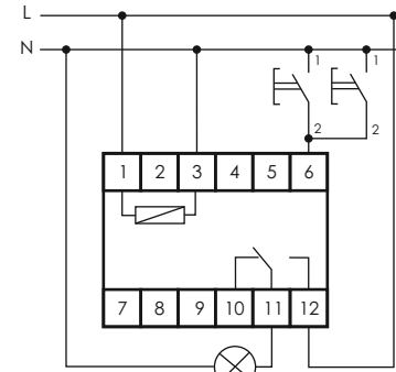
Схема подключения с управлением от нуля "N".
