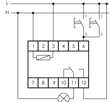
Схема подключения с управлением от фазы "L".
