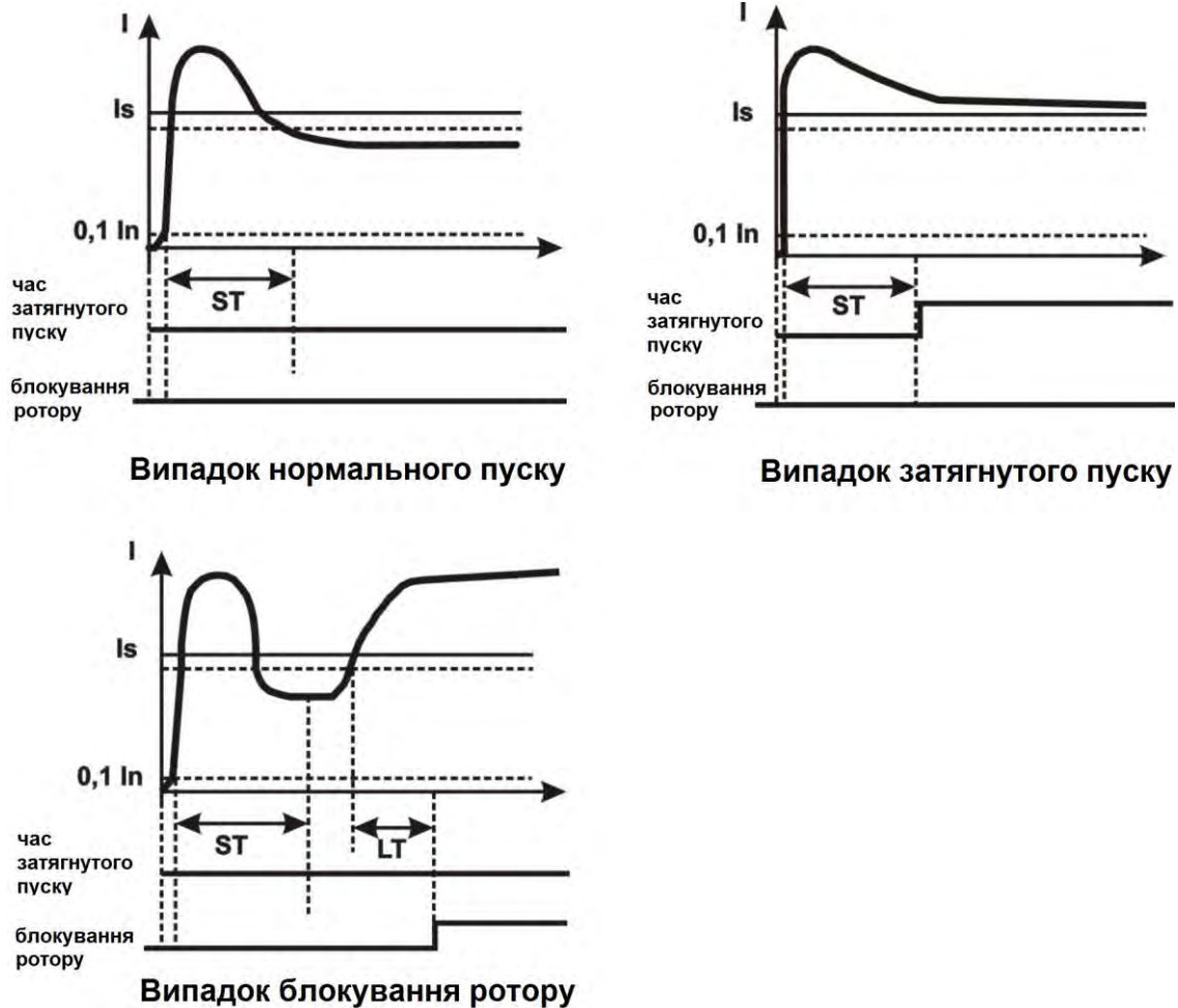
Рисунок 3.3 - Зягнутий пуск та блокування ротора
