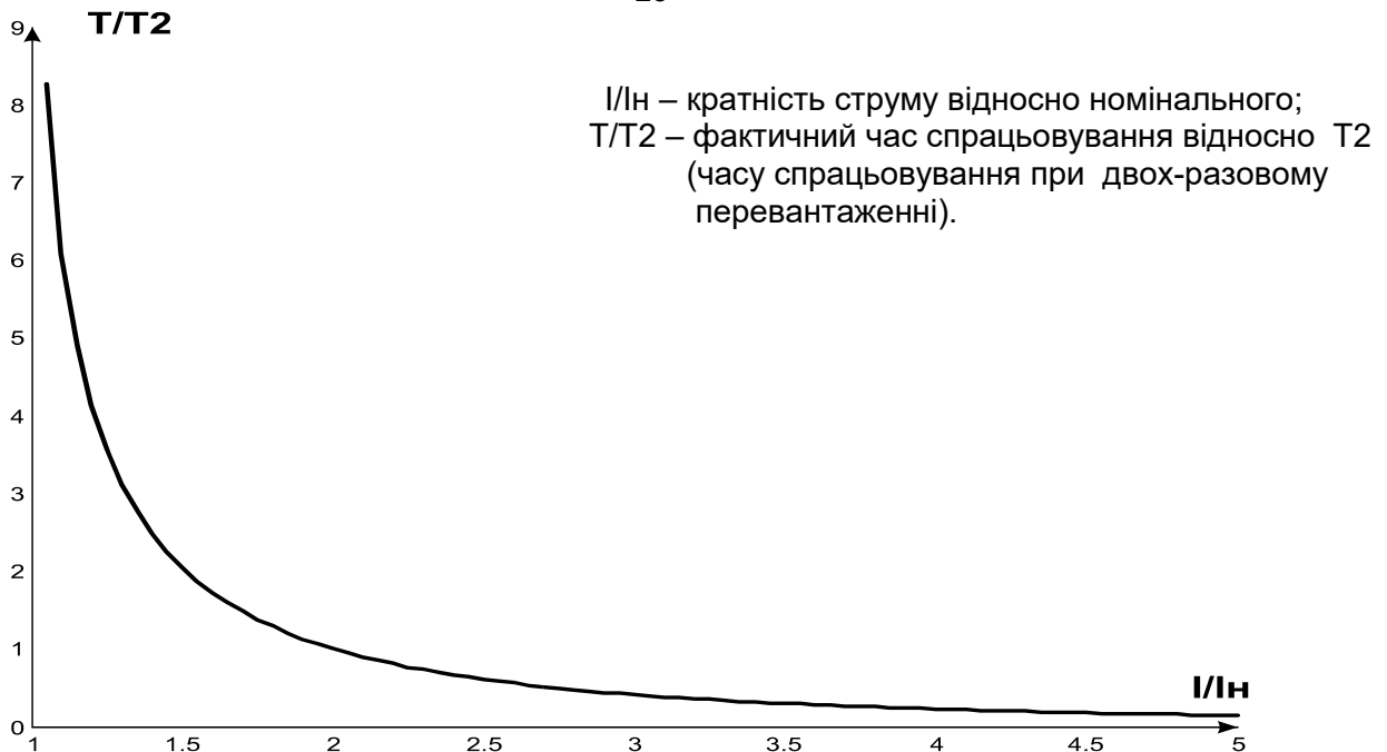
Рисунок 3.4 - Струмо-часова характеристика
