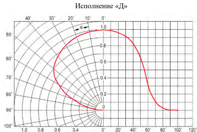
Рисунок 7 Тип КСС
