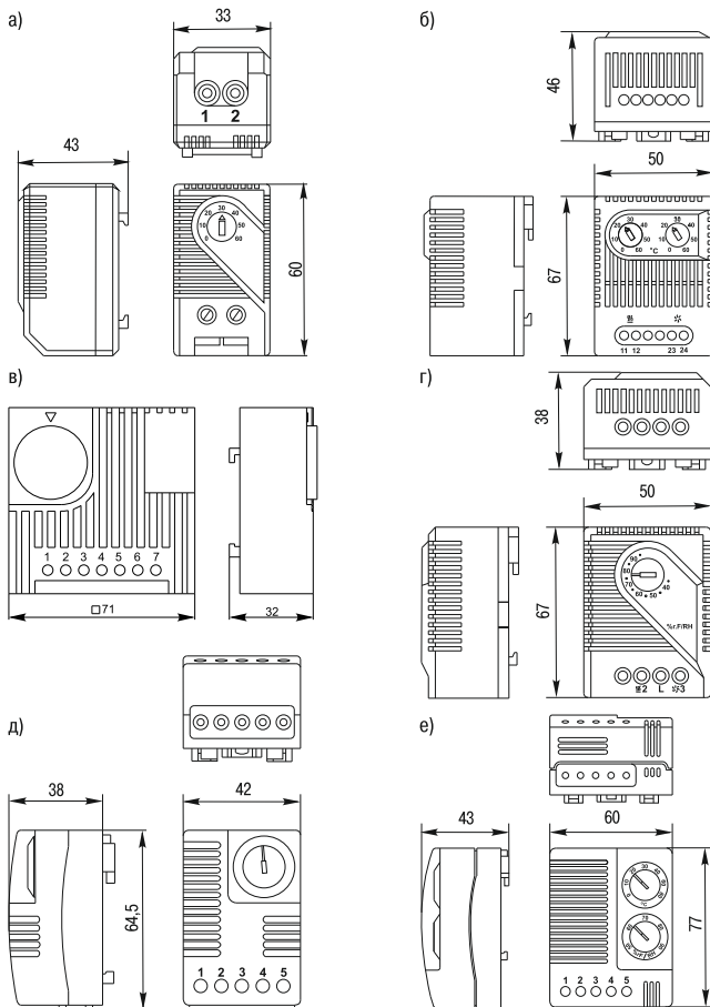
Рисунок 1 – а) термостаты УККт NO и NC; б) термостат двухканальный УККт; в) термостат УККт NO/NC; г) гигростат механический УККт; д) гигростат электронный УККт; е) гигротерм УККтг
