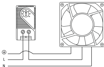
Пример подключения
