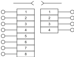
Рисунок 3 – Электрическая схема розеток компьютерная/телефонная серии КВАРТА
