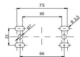
Установочні розміри
