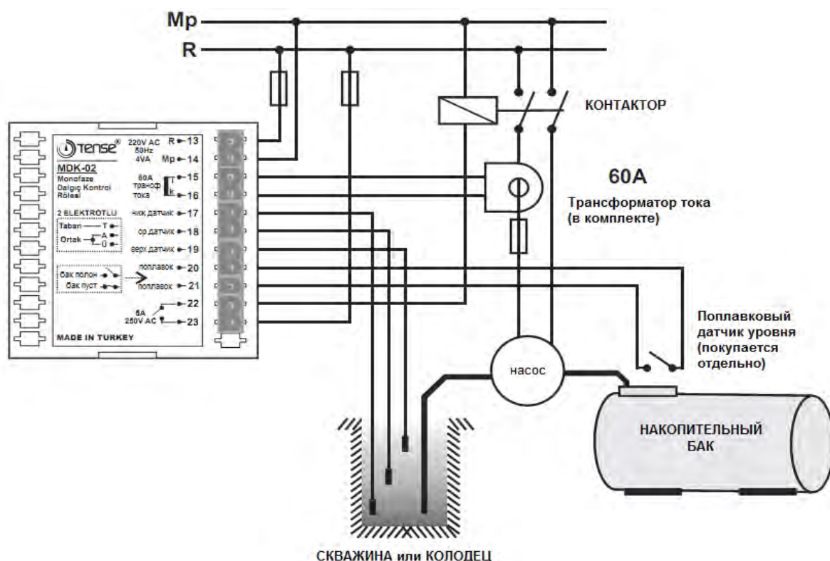
Рис.1. Схема подключения
