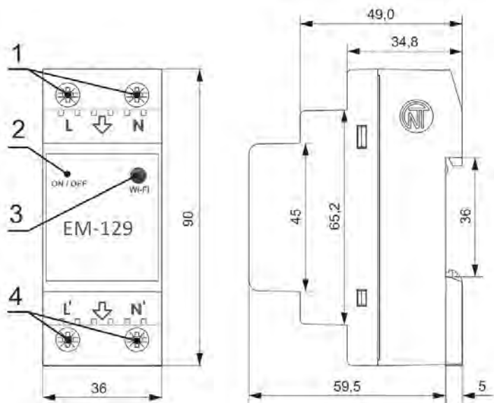
Рисунок 1 – Органы управления, габаритные и установочные размеры EM-129
