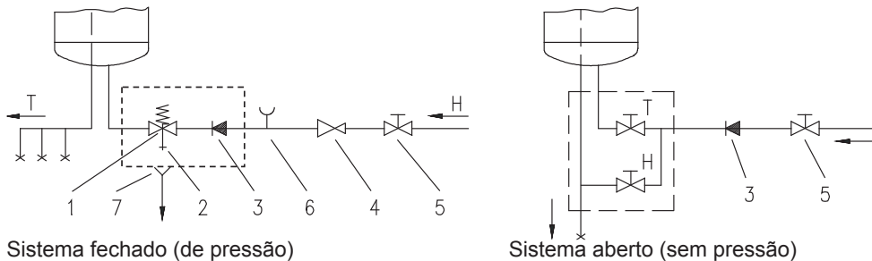
Sistema fechado (de pressão)
