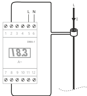
Версія з трансформатором струму
