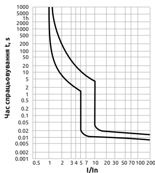
Характеристика С (1-63А)
