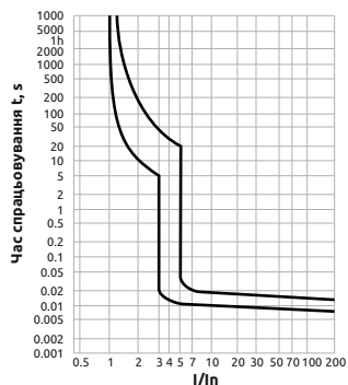
Характеристика В (1-63А)
