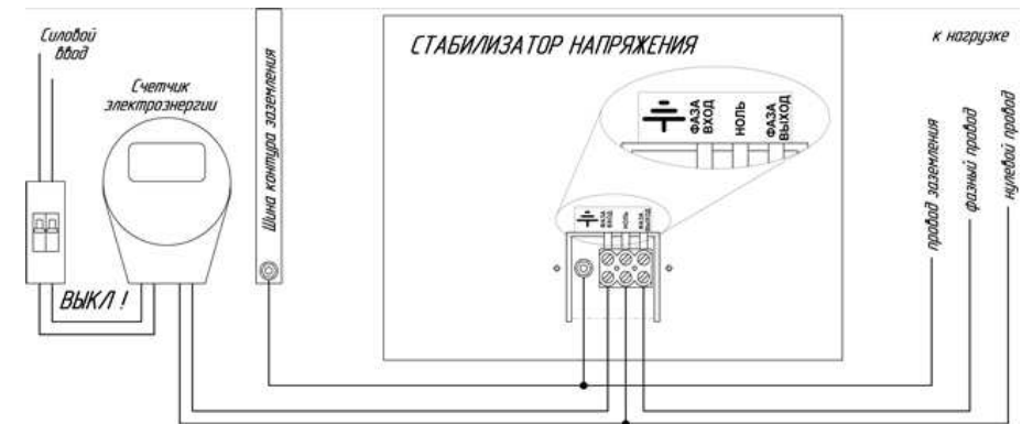
Рисунок 2. Рекомендуемая схема подключения стабилизатора к сети.
