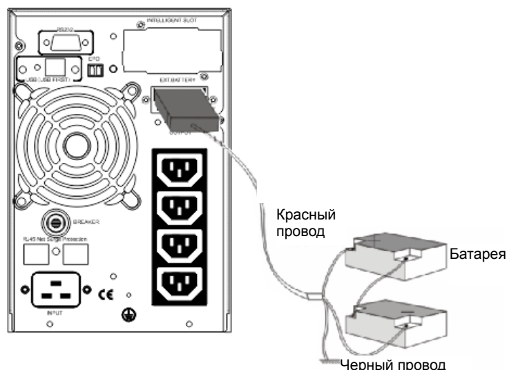
FIG.7 подключение батареи
