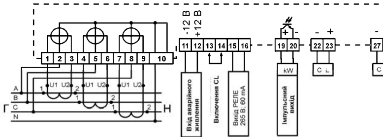
Рисунок 1 - Схема підключення лічильника
