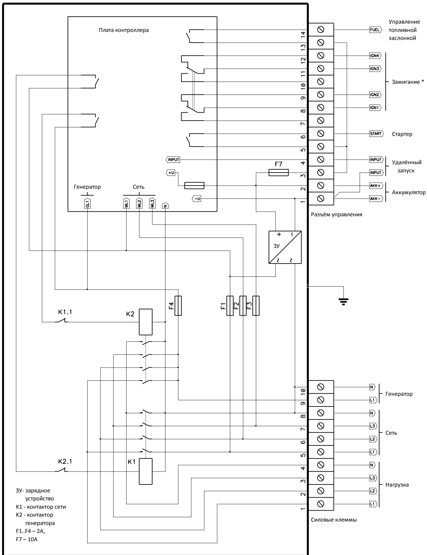
Рис 6.2. Пример схемы подключения контроллера AVR313ME.
