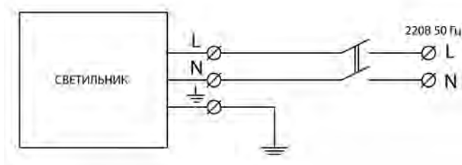
Рисунок 2 Схема подключения светильника
