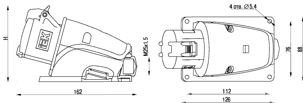
Рисунок А.5 – Габаритные размеры соединителей типа ССИ-233, ССИ-234, ССИ-235/ Figure A.5 – Overall dimensions of couplers SSI-233, SSI-234, SSI-235 type
