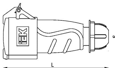
Рисунок А.4 – Габаритные размеры соединителей типа ССИ-213, ССИ-214, ССИ-215, ССИ-223, ССИ-224, ССИ-225/ Figure A.4 – Overall dimensions of couplers SSI-213, SSI-214, SSI-215, SSI-223, SSI-224, SSI-225
