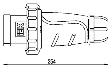
Рисунок А.2 – Габаритные размеры соединителей типа ССИ-033, ССИ-034, ССИ-035/ Figure A.2 – Overall dimensions of couplers SSI-033, SSI-034, SSI-035 type
