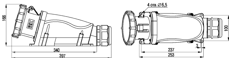
Рисунок А.9 – Габаритные размеры соединителей типа ССИ-145/ Figure A.9 – Overall dimensions of couplers SSI-145 type
