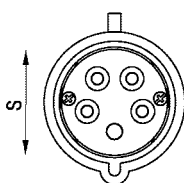
Рисунок А.1 – Габаритные размеры соединителей типа ССИ-013, ССИ-014, ССИ-015, ССИ-023, ССИ-024, ССИ-025/ Figure A.1 – Overall dimensions of couplers SSI-013, SSI-014, SSI-015, SSI-023, SSI-024, SSI-025 type
