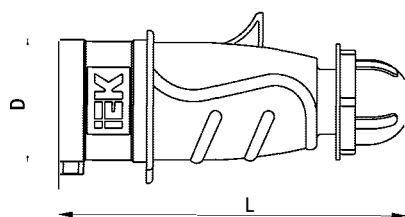
Рисунок А.1 – Габаритные размеры соединителей типа ССИ-013, ССИ-014, ССИ-015, ССИ-023, ССИ-024, ССИ-025/ Figure A.1 – Overall dimensions of couplers SSI-013, SSI-014, SSI-015, SSI-023, SSI-024, SSI-025 type
