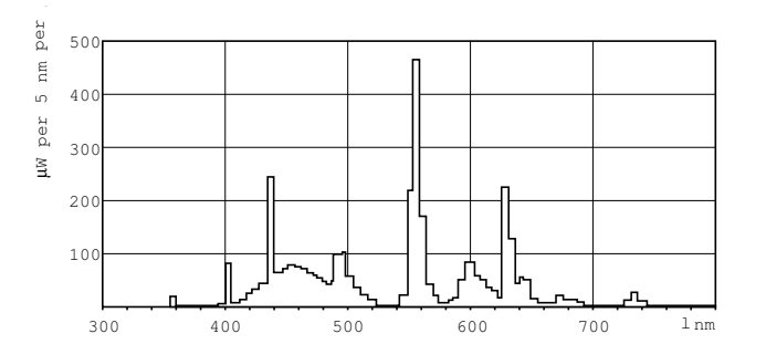
Цвет излучения /865
