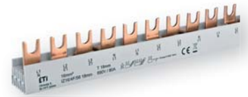
IZ16/4F/56
