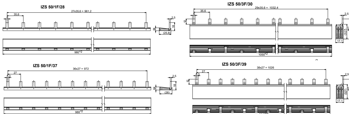
IZS 50/3F/39
