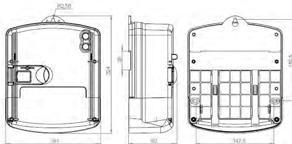
Рисунок 2 - Габаритні і передувальні розміри лічильника
