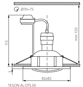
TESON AL-DTL50
