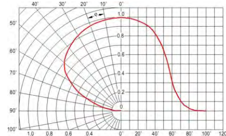
Рисунок 3 Тип КСС в исполнении «Д»
