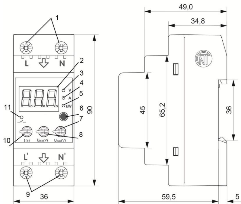
Рисунок 1 – Органы управления и габаритные размеры РН-263t
