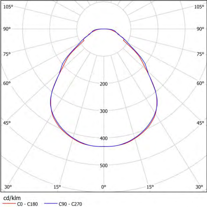
Рисунок 4 Типы КСС
