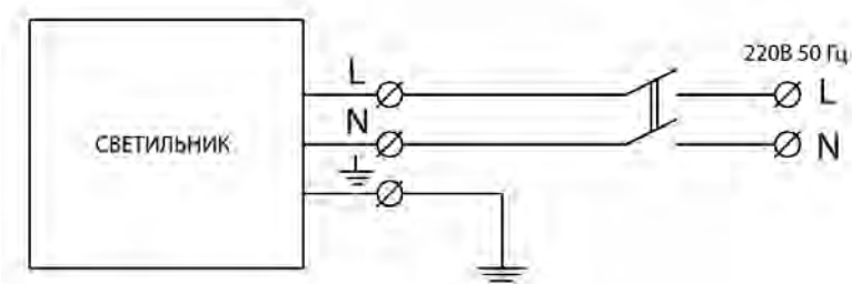
Рисунок 3 Схема подключения светильника
