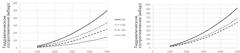
Графики потери напора воды (CWH Elitec 200.2-1500.2)
