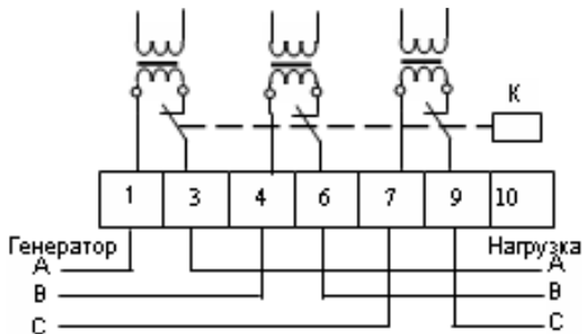
Рисунок 3.11 - Схемы подключения реле
