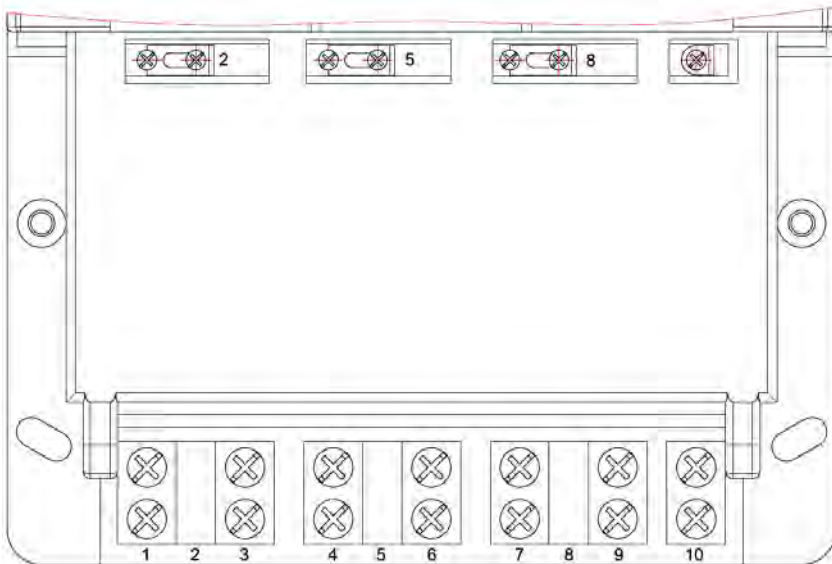
е) - обозначение контактов зажимов счетчика CE 303 S34
