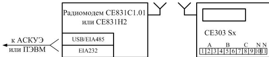
Рисунок 3.7 - Схема подключения счетчика
