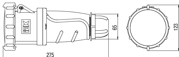
Рисунок 5 – Габаритные размеры соединителей типа ССИ-233, ССИ-234, ССИ-235
