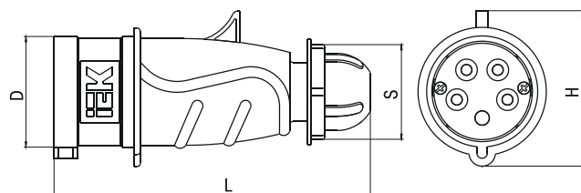
Рисунок 1 – Габаритные размеры соединителей
