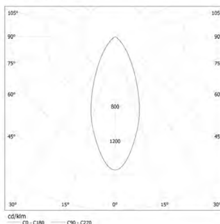
KANLUX S.A. (kat 28251) ARME LED O 5W-WW / LDC (Polar)
