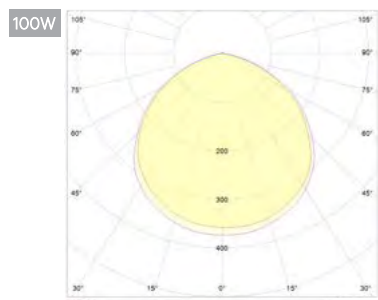
Кут розсіювання 120° Angle scattering
