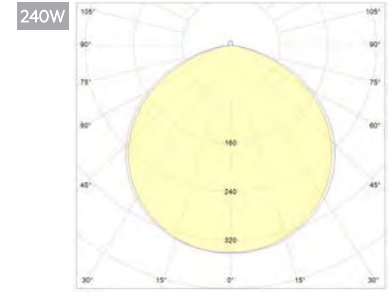
Кут розсіювання 120° Angle scattering
