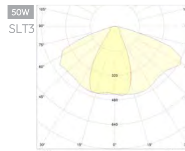
Кут розсіювання 120° Angle scattering
