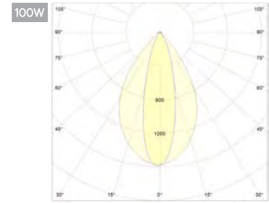
Кут розсіювання 30*70° Angle scattering
