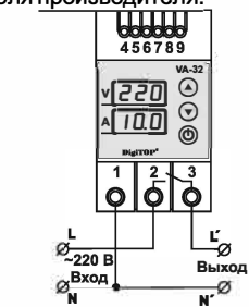
Схема подключения
