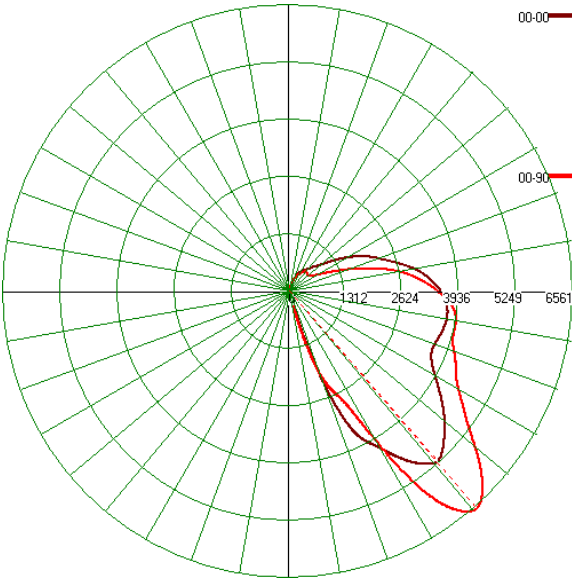
Рисунок 3 Типы КСС
