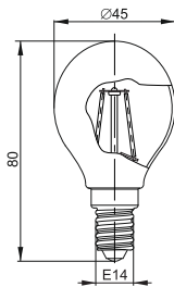
Рисунок 4 – Лампа LED-G45 серия 360° 5 Вт, 7 Вт цоколь E14
