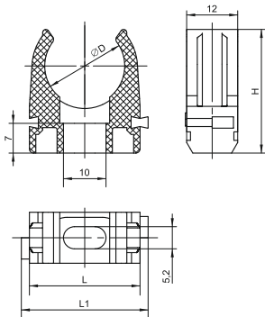
Рисунок 1 – Держатель с защёлкой
